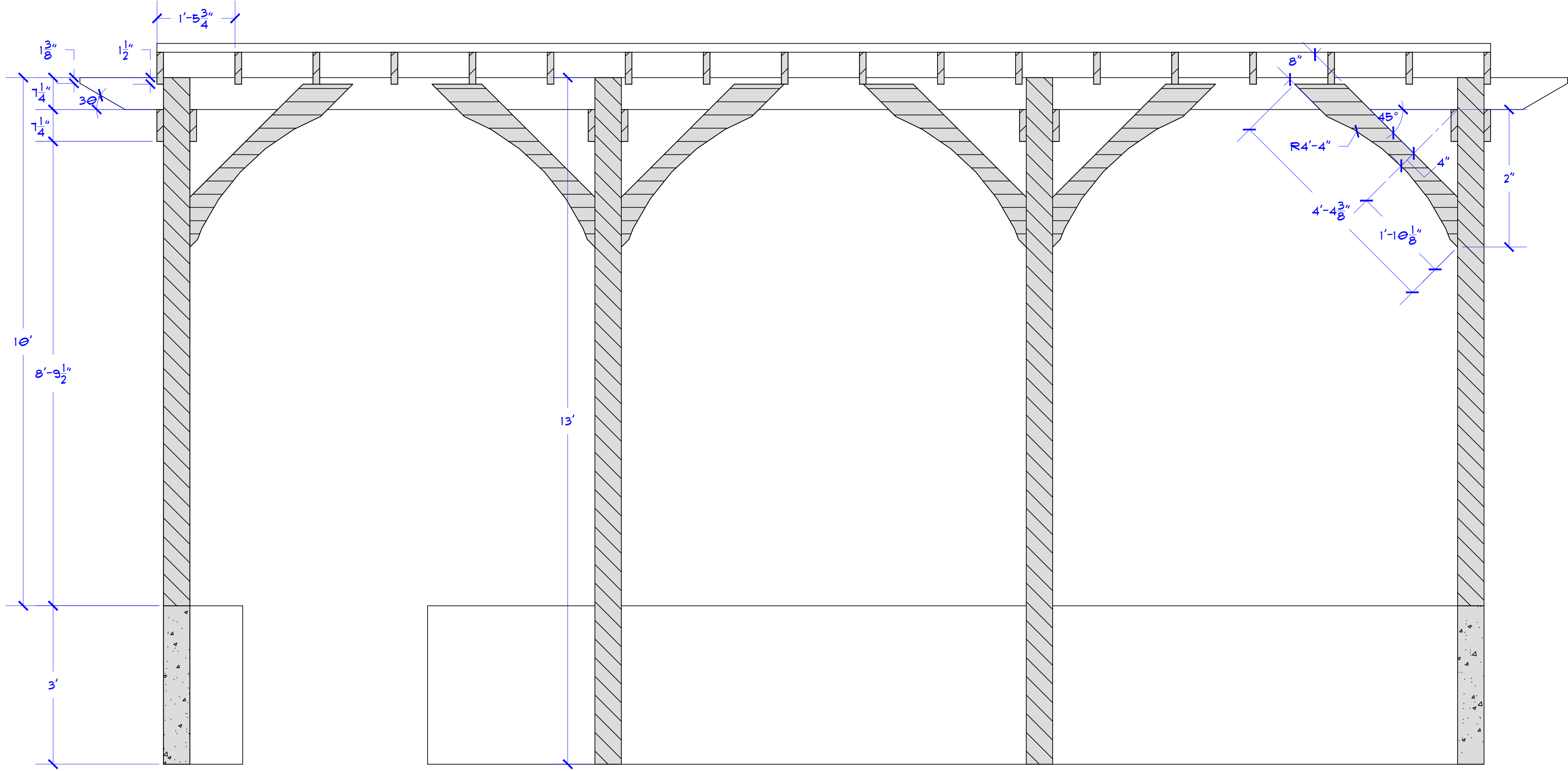
2A SECTION SCALE: 3/4" = 1'
